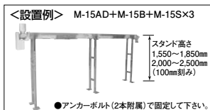
●アンカーボルト(2本付属)で固定して下さい。 モミトップスタンド M-10S/M-15S
