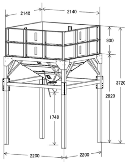
●HBK-26S寸法図
