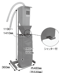
吸太郎用紙袋スタンド KQ-S
