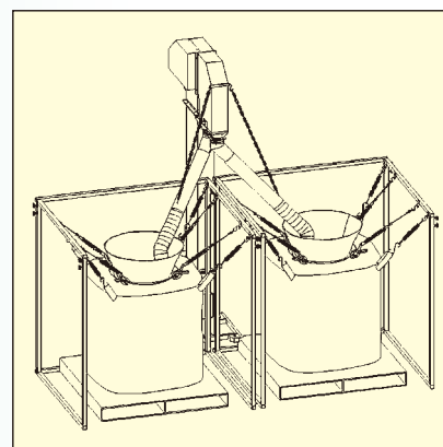
フレコンバックスタンド2台配置図
