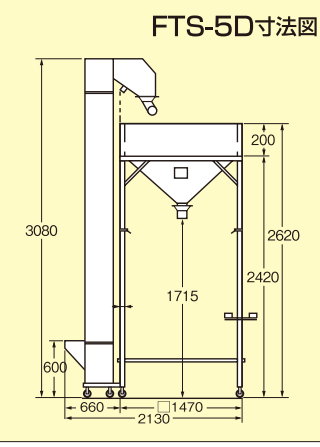
FTS-5D寸法図
