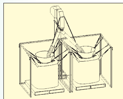
フレコンバックスタンド2ヶ配置図
