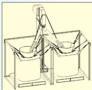
フレコンバック スタンド 2ヶ配置図
