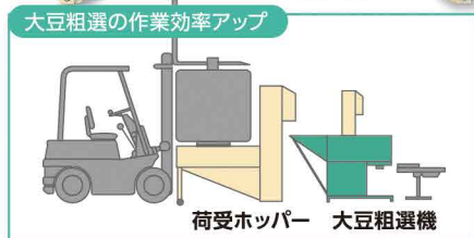
ホッパーシャッターはレバーにより調整可能
