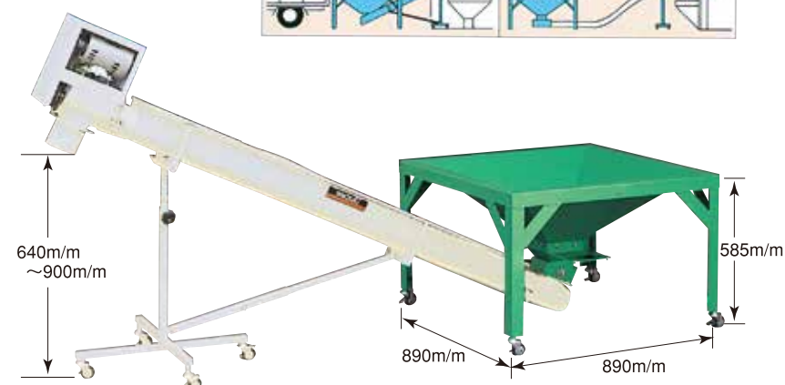
※籾入ホッパー3H+ラセコンU-20A
