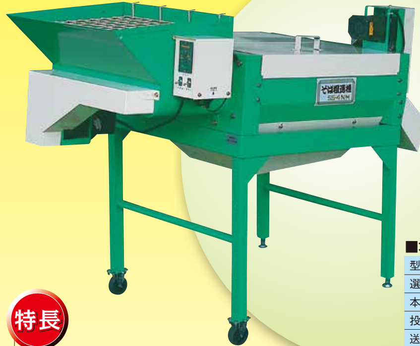
送りラセンによって張込み量を調整できます。
