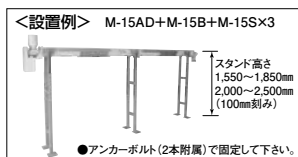
アタッチメント (モミトップスタンドM-10S(M-10用)・M-15S(M-15用))
