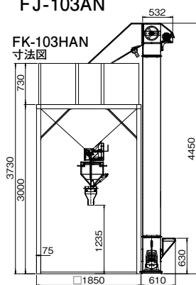
フレコンスケール FJ-103AN
