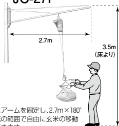
玄米キャッチャー ジブクレーンタイプ JC-27P
