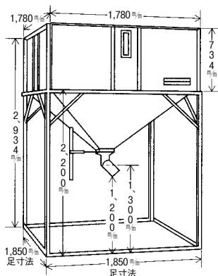
●HSK-15寸法図
