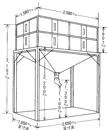
●HB-27寸法図
