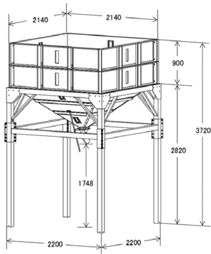
●HBK-26S寸法図
