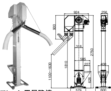
フレコン用昇降機 FSH-27A
