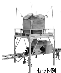
セット例 SA-10+SB-10
