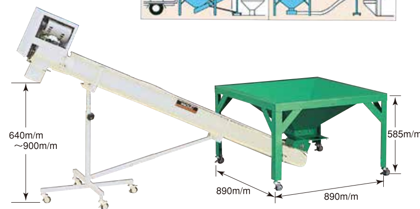
※粉入ホッパー3H+ラセコンU-20A
